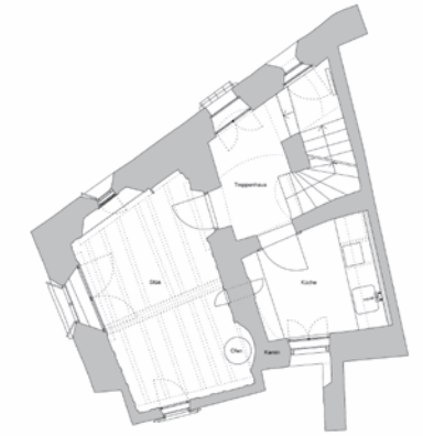
Grundriss 1. Obergeschoss
